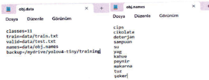
Şekil 4. Sınıf ve veri yolu tanımları: obj.names ve obj.data dosyaları
