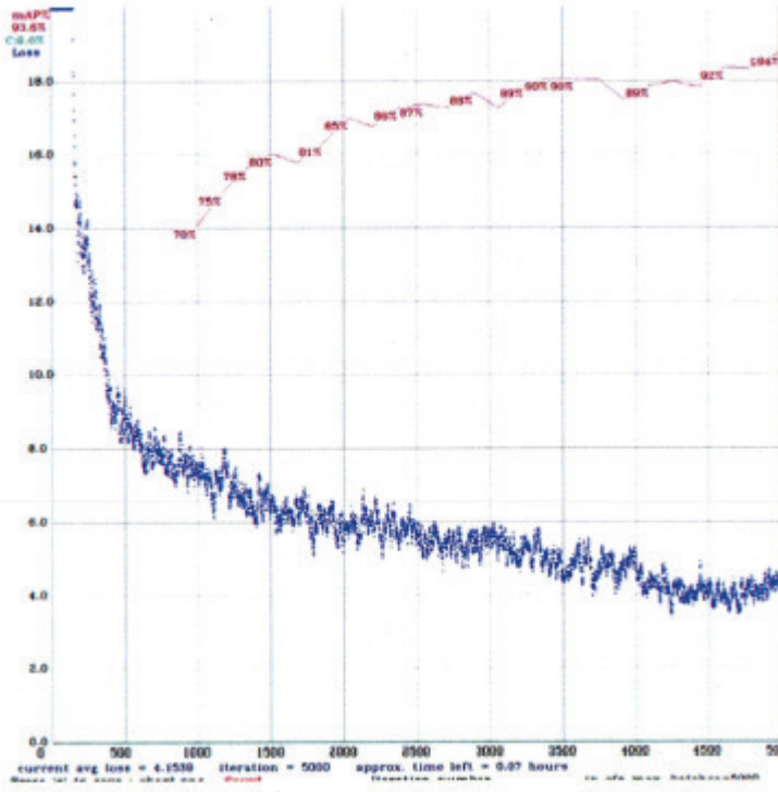
Şekil 7. YOLO eğitim grafiği.
